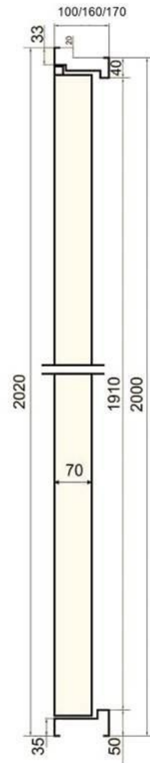
Zvislý rez
