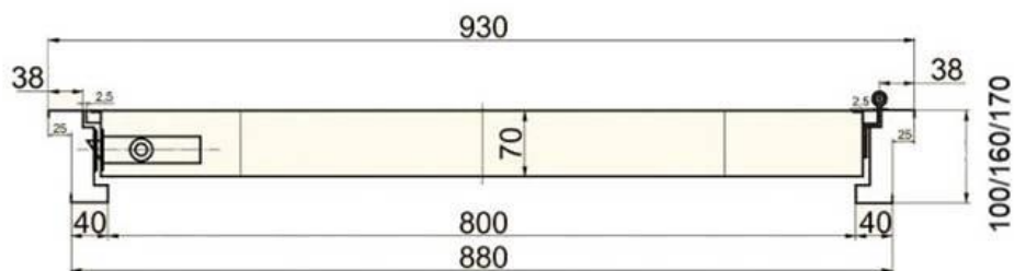
Vodorovný rez
